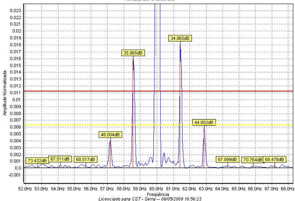
Figura 3. Gráfico característico de uma condição de barra quebrada.
