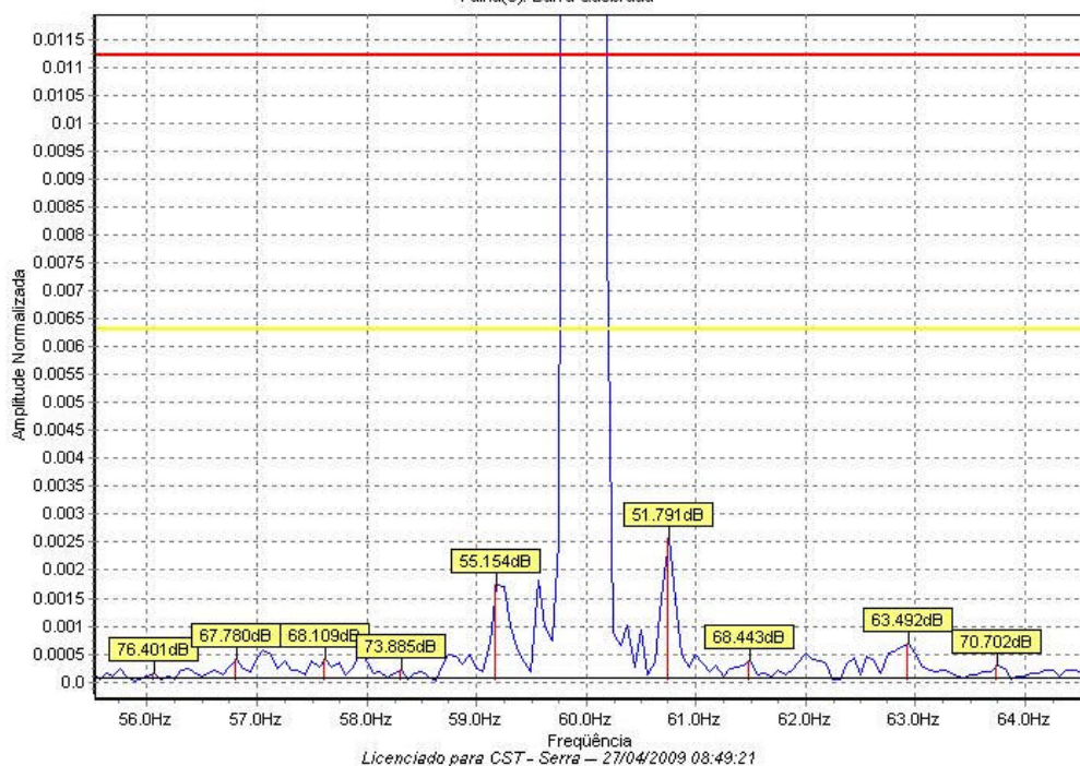
Figura 11 - Gráfico registrado após o conserto das barras quebradas.
