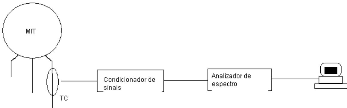
Figura 1. Sistema básico para análise espectral da corrente
