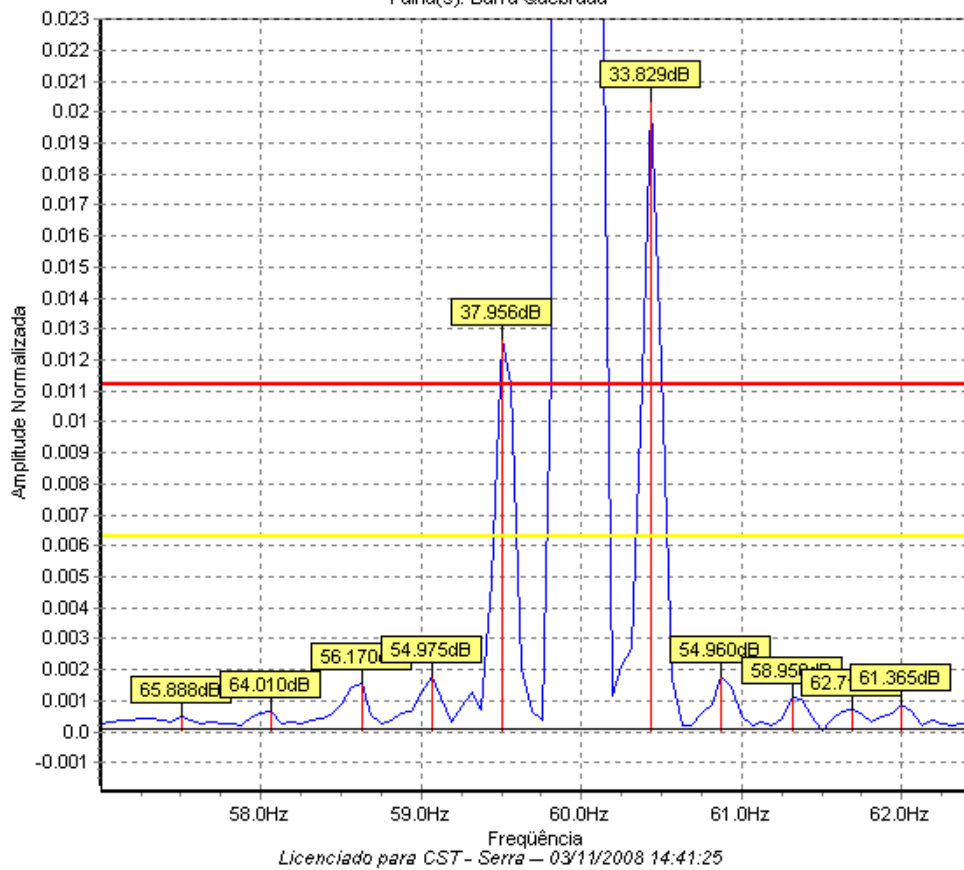
Figura 4. Gráfico da falha.
