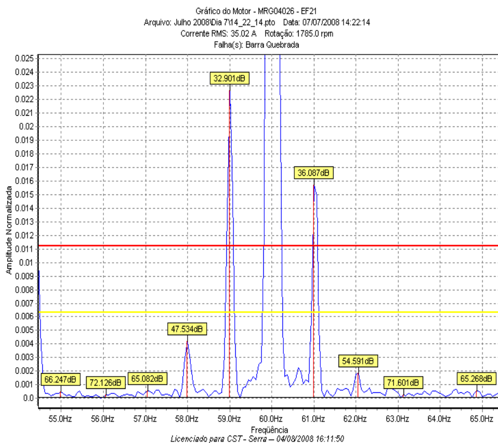
Figura 8 – Gráfico da falha.
